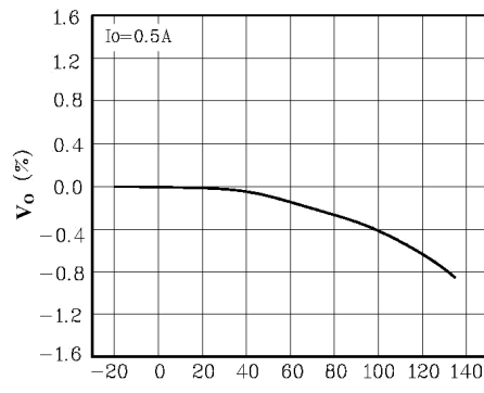
V_O - T_a
