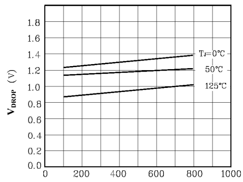
V_{DROP} - I_O
