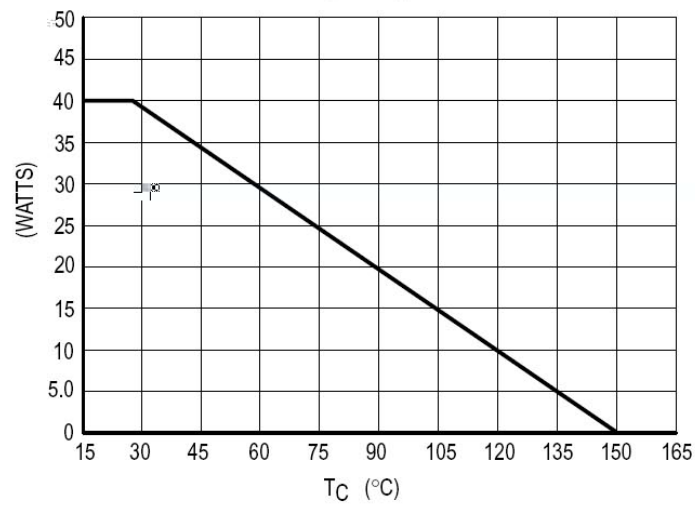
P_D - T_C
